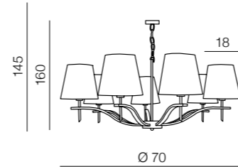
Princessa 7 AZ0725 E14 7x 40W metal/chrome/fabric
